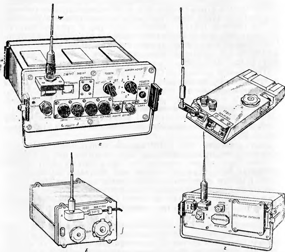
Рис. 12. Комплекс малогабаритных разведывательно-сигнализационных средств: а — прибор контроля; б — малогабаритное разведывательно-сигнализационное устройство; в — устройство приема информации; г — ретранслятор
